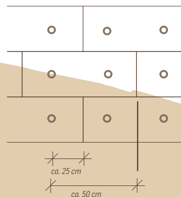
Schraubenabstand, Plattenabstand
