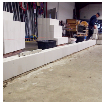
Setzen der Steine ohne großen Aufwand, zügiges Mauern ohne Stoßfugenvermörtelung
