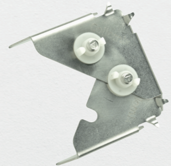
Ausnivellieren der Anlegehilfen und auflegen des Ansetzmörtels
