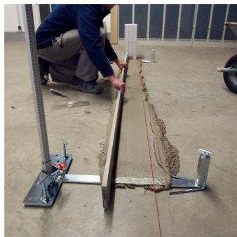
Planes Abziehen des Mörtelbetts in Längs- und Querrichtung
