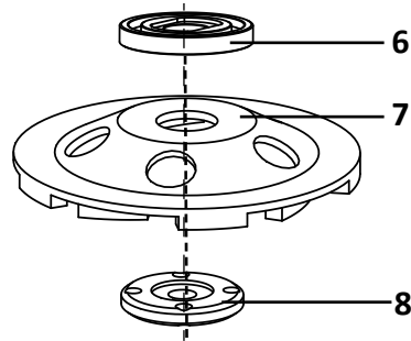
Montering av koppskiven
