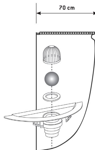
Montage der Geruchssperre MEASTOP für MEAMULTINORM, Tiefe 70 cm
