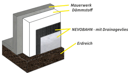
EINSATZ ALS GRUNDMAUERSCHUTZ
