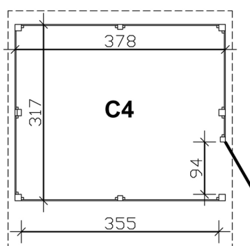
Grundriss Abstellraum C4
