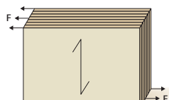
K f_{v,90,edge} hochkant, rechtwinklig♦♦
