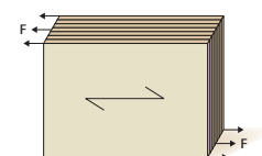
J f_{v,0,edge} und G_{0,edge} hochkant, parallel♦
