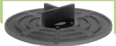
Abbildung 2: gummierte Volfiplatte VP-GKU 0/00 als verbreiterte Auflagefläche für FK-BT
