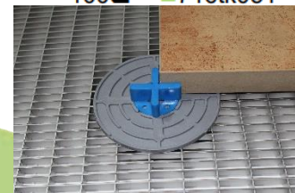
Abbildung 4: FK-B mit VP-GKU auf Gitterrost verlegt
