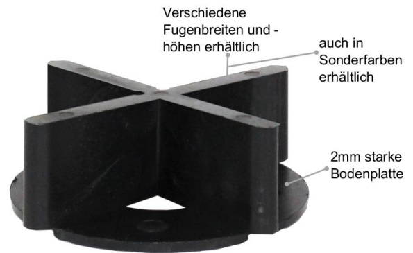
Abbildung 1: Fugenkreuz mit Bodenplatte, Farbe: schwarz
