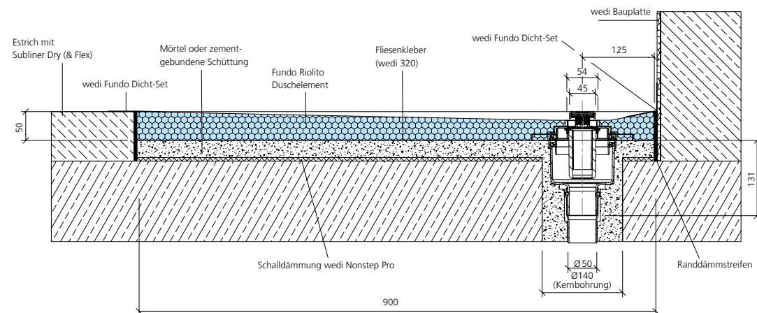
wedi Fundo Rinnenablauf senkrecht, DN 50, Estrichfußboden
