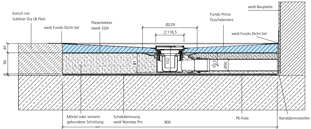
wedi Fundo Punktablauf waagerecht, DN 50, Estrichfußboden
