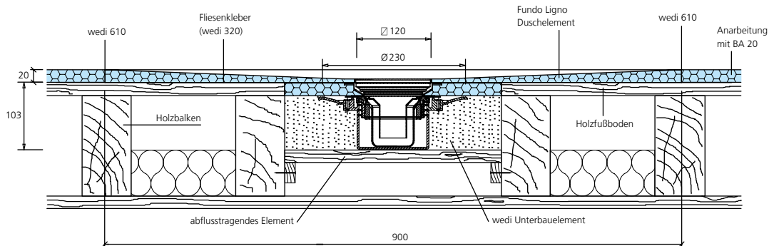
wedi Fundo Punktablauf waagrecht, DN 50, auf Holzbalkendecke
