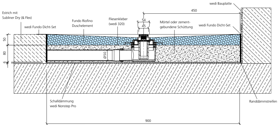
wedi Fundo Rinnenablauf waagrecht, DN 50, Estrichfußboden
