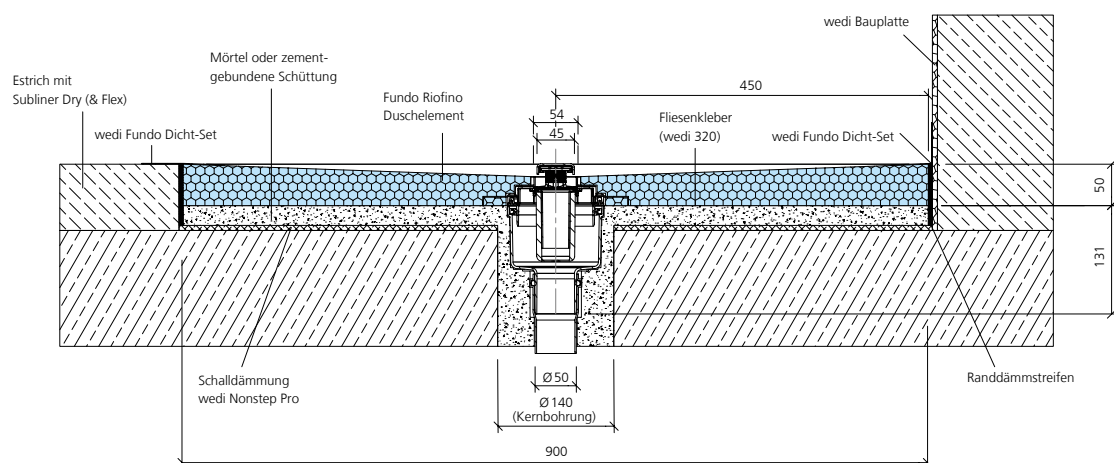
wedi Fundo Rinnenablauf senkrecht, DN 50, Estrichfußboden
