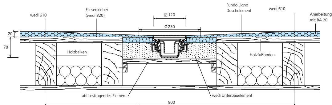
wedi Fundo Punktablauf Mini Max, DN 40, auf Holzbalkendecke
