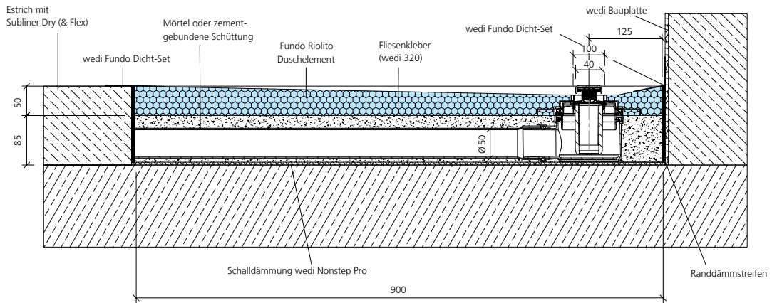
wedi Fundo Rinnenablauf waagrecht, DN 50, Estrichfußboden
