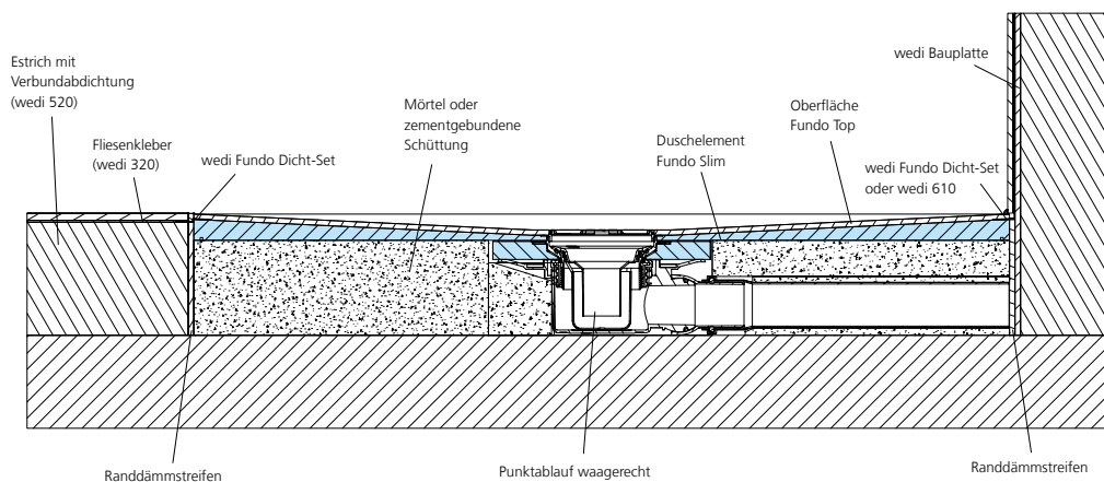
wedi Fundo Punktablauf waagrecht, DN 50, in Estrichfußboden
