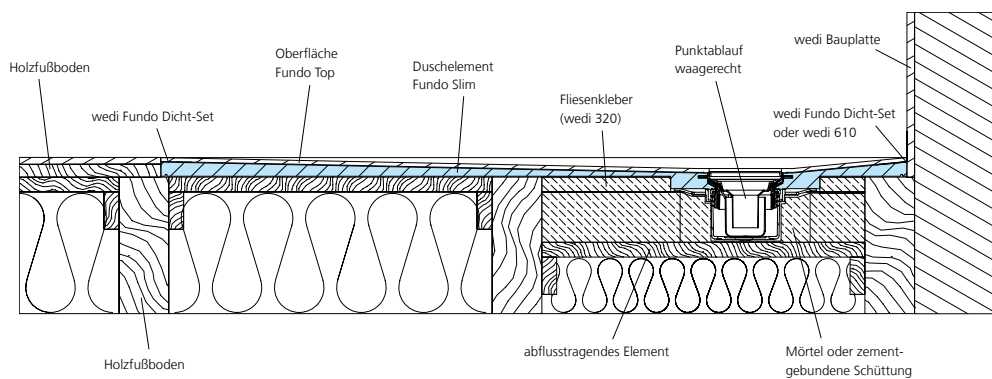
wedi Fundo Punktablauf waagrecht, DN 50, in Holzbalkendecke
