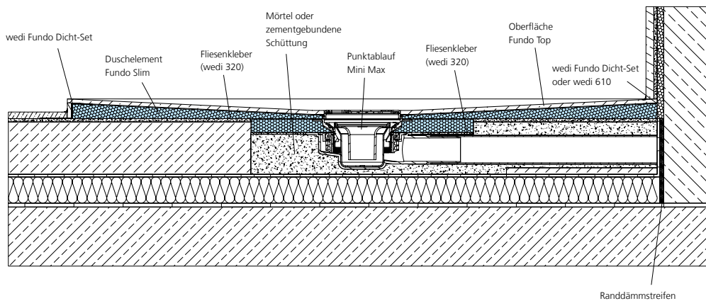
wedi Fundo Punktablauf Mini Max, DN 40, auf Estrichfußboden
