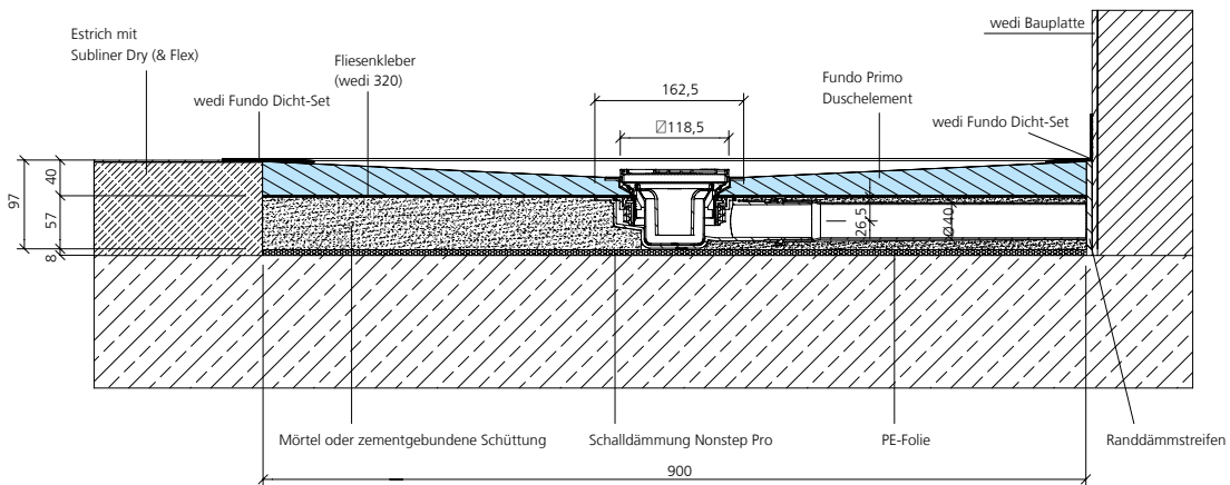
wedi Fundo Punktablauf Mini Max, DN 40, Estrichfußboden
