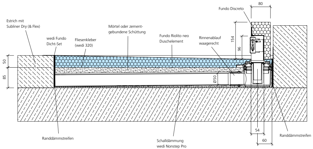
Fundo Discreto, Wandablauf, DN 40, Estrichfußboden
